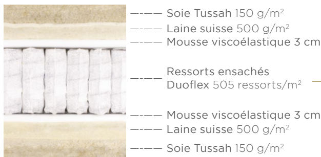
Ressort Duoflex support progressif longue durée
